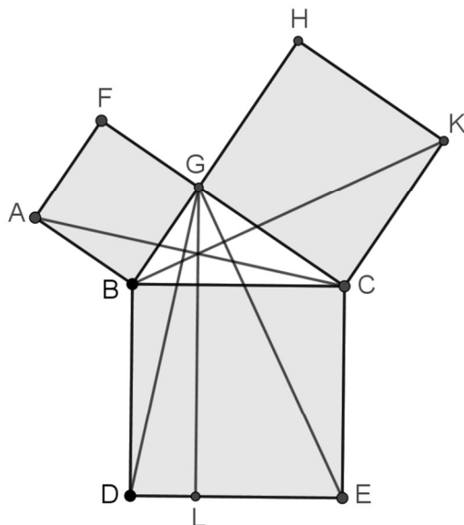
Figura 3.9 – O Teorema de Pitágoras.
