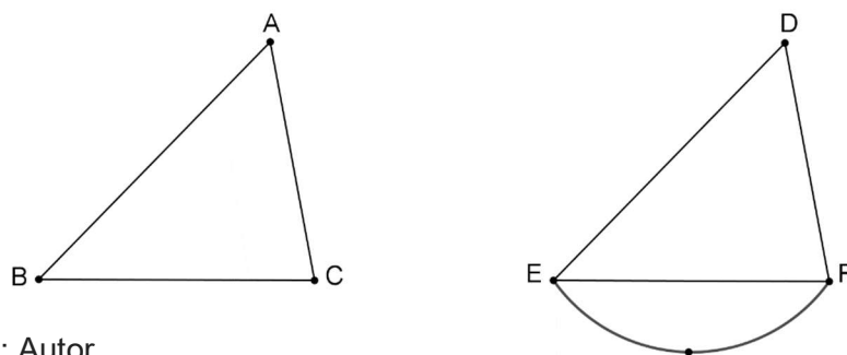
Figura 3.4 – Demonstração do caso LAL – Lado-Ângulo-Lado.
