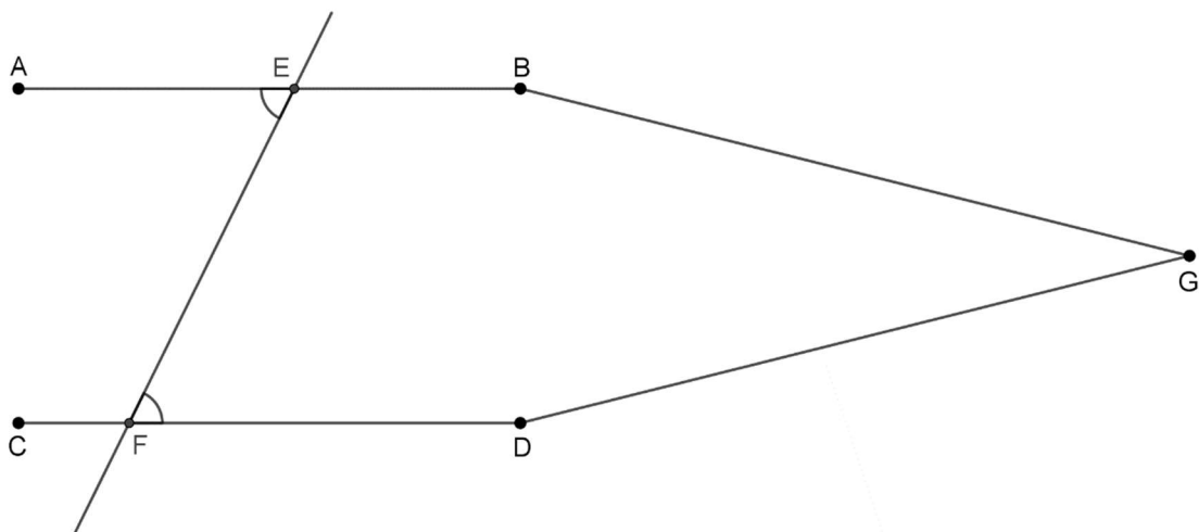
Figura 2.11 – Retas paralelas, uma aplicação do V axioma.
