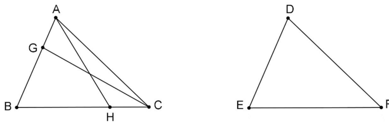
Figura 3.6 – Demonstração do caso ALA – Ângulo-Lado-Ângulo.
