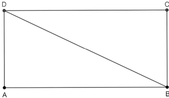
Figura 2.10 – Gráfico II de Nasiraddin.
