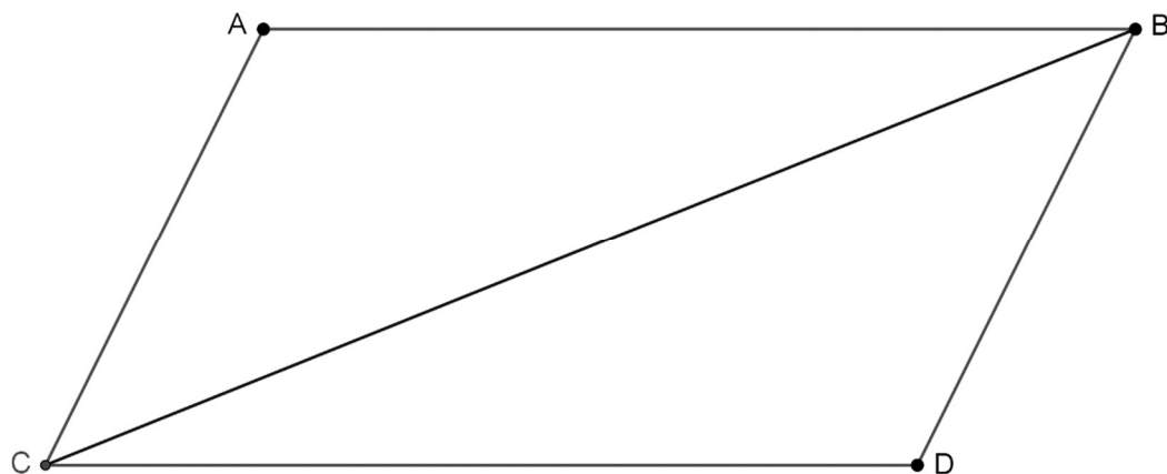
Figura 3.3 – Paralelogramos, lados e ângulos opostos iguais.
