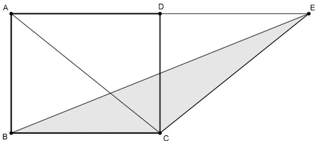
Figura 3.11 – Paralelogramo sendo o dobro de um triângulo.
