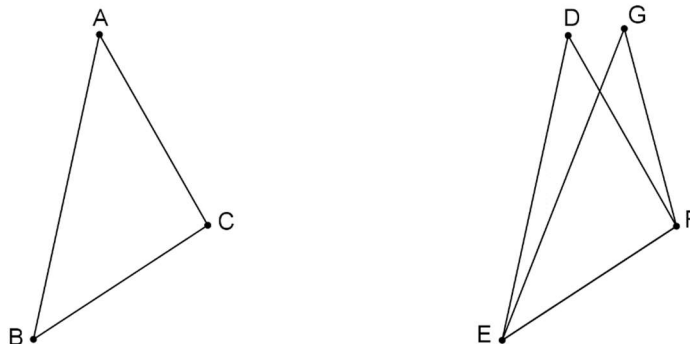
Figura 3.5 – Demonstração do caso LLL – Lado-Lado-Lado.
