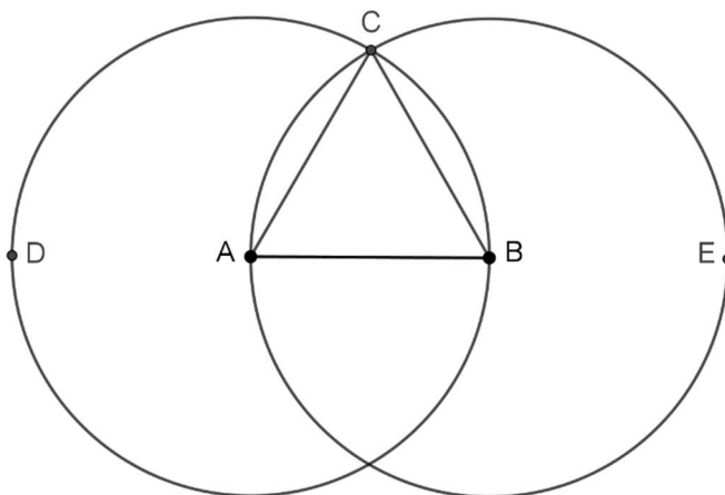
Figura 1.1 – Construção de um triângulo equilátero.
