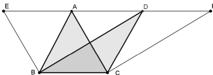
Figura 3.2 – Triângulos de mesma base e entre paralelas.
