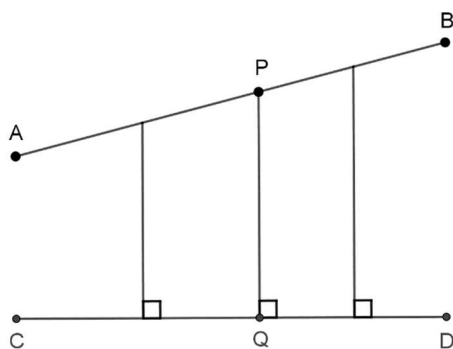
Figura 2.9 – Suposição de Nasiraddin-Tusi.
