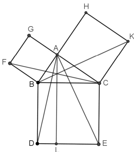
Figura 3.10 – Demonstração do Teorema de Pitágoras.
