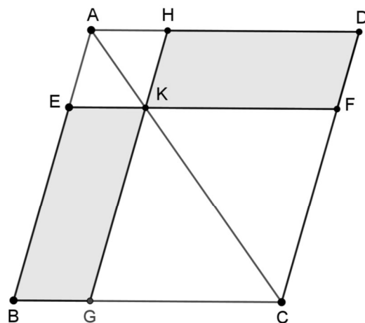
Figura 3.7 – Complementos dos paralelogramos.
