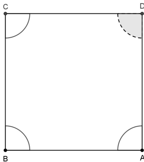
Figura 2.12 – Teoria das linhas paralelas
