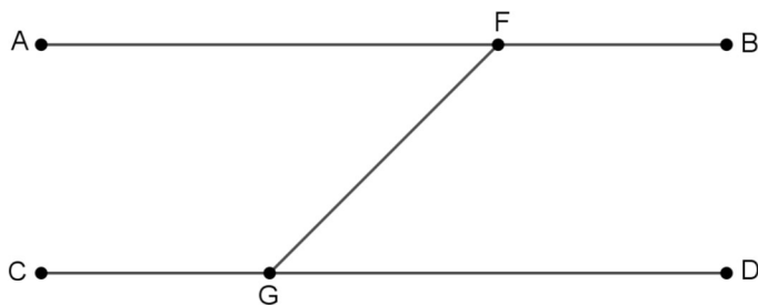
Figura 2.6 – Retas paralelas de Ptolomeu.
