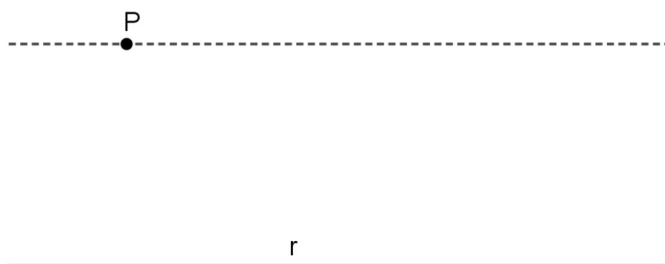
Figura 2.7 – Axioma das paralelas.
