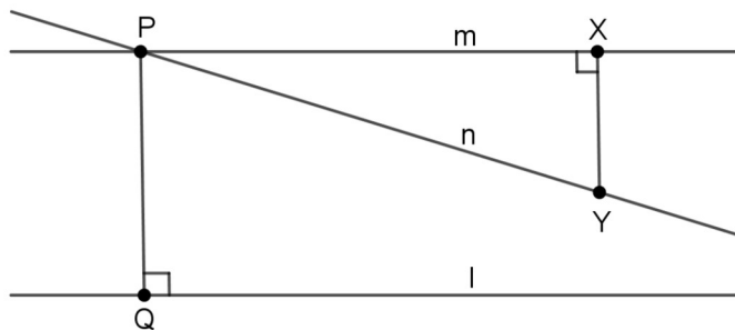
Figura 2.8 – Retas paralelas segundo Proclo.
