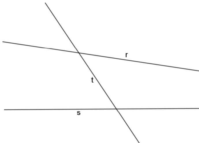
Figura 2.5 – O quinto axioma.
