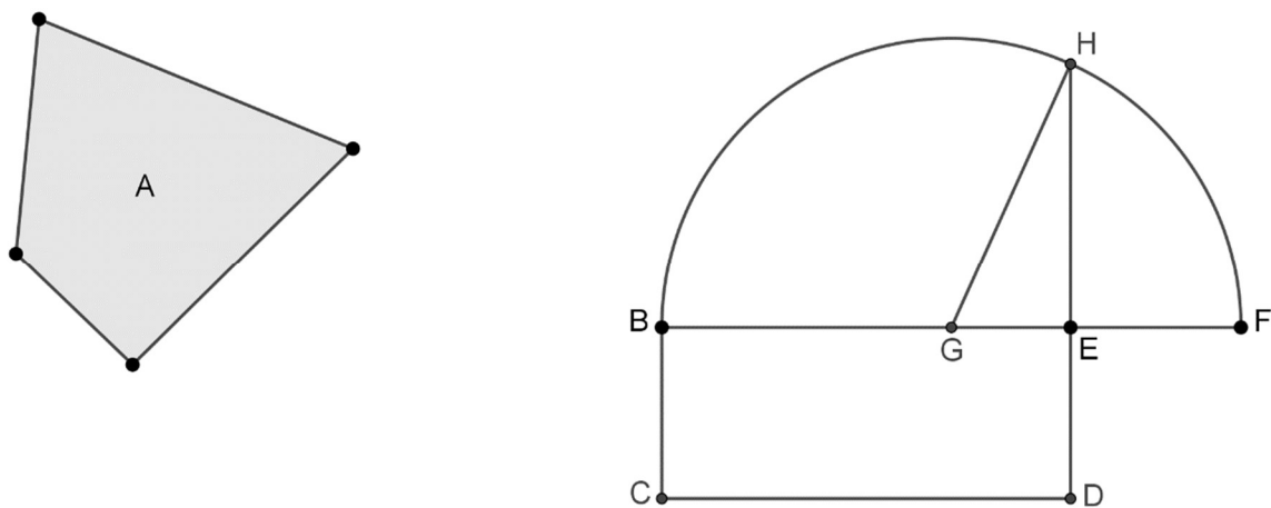
Figura 3.14 – Quadratura de uma figura plana poligonal.
