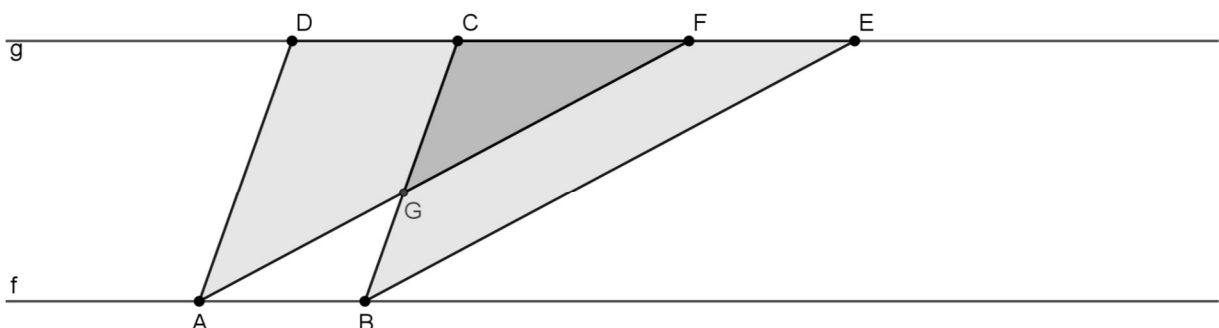
Figura 3.1 – Paralelogramos de mesma base e entre paralelas.
