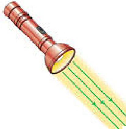
Figura 4: Raios de luz representados por retas orientadas.
