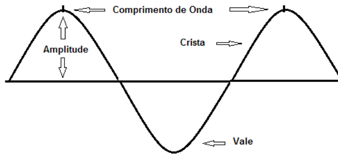
Figura 40 : Elementos de uma onda.
