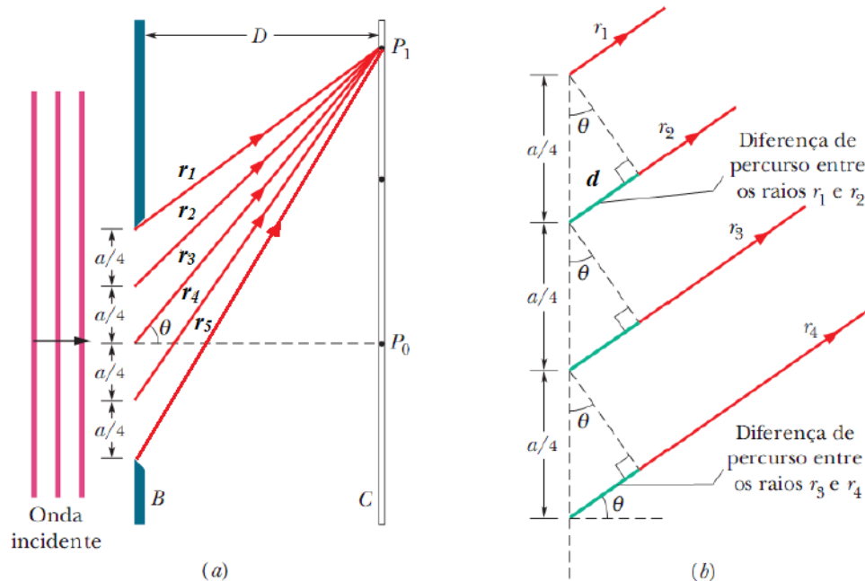
Figura 15 : (a) os raios provenientes da extremidade superior de quatro regiões de largura a/4 sofrem interferência destrutiva no ponto p_1 . (b) para d \gg a , podemos supor que os raios r_1, r_2, r_3, r_4 e r_5 são aproximadamente paralelos e fazem um ângulo \theta com o eixo central.
