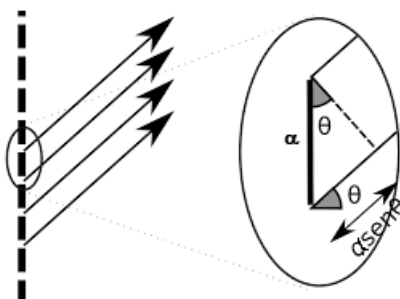
Figura 56: Múltiplas fendas simplificadas.
