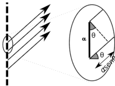
Figura 19: Múltiplas fendas simplificadas.
