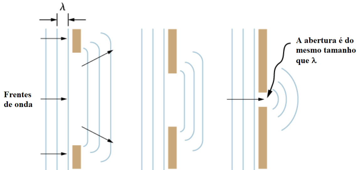
Figura 43: Frentes de onda projetada em uma fenda. À medida que a fenda diminui, fica mais evidente o efeito de difração.
