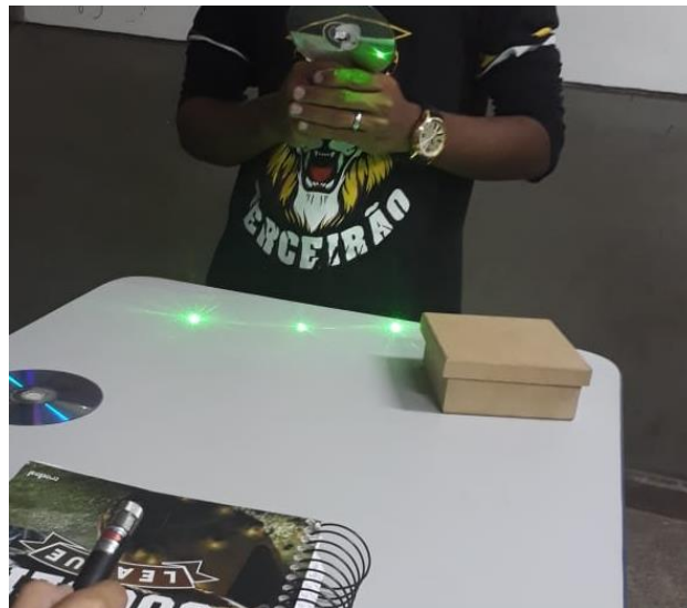
Figura 65 - Experimento demonstrando os feixes espaçados produzidos pela rede
