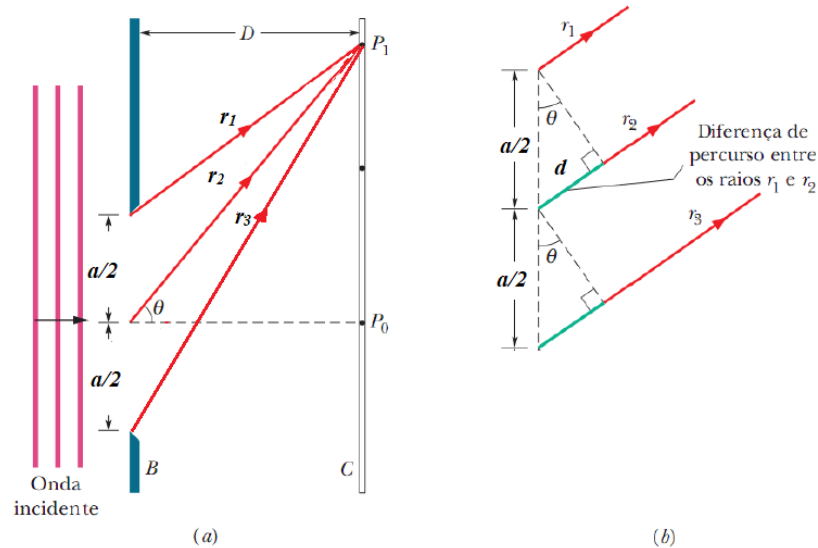
Figura 14 : (a) Os raios provenientes da extremidade superior de duas regiões de largura a/2 sofrem interferência destrutiva no ponto p_1 . (b) para d \gg a , podemos supor que os raios r_1 e r_3 são aproximadamente paralelos e fazem um ângulo \theta com o eixo central.
