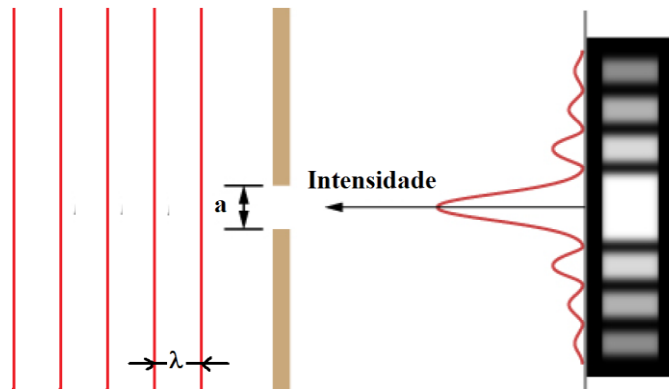
Figura 50 : Padrão de difração e interferência de fenda única. A luz monocromática que passa através de uma única fenda tem um máximo central, o mais brilhante, e máximos secundários (de intensidades menores) e escuros de cada lado.
