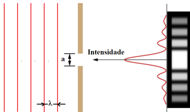
Figura 13 : Padrão de difração e interferência de fenda única. A luz monocromática que passa através de uma única fenda tem um máximo central, o mais brilhante, e máximos secundários (de intensidades menores) e escuros de cada lado.
