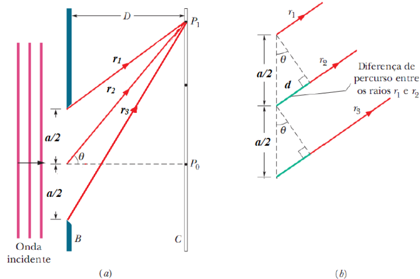
Figura 51 : (a) Os raios provenientes da extremidade superior de duas regiões de largura a/2 sofrem interferência destrutiva no ponto p_1 . (b) para d \gg a , podemos supor que os raios r_1 e r_3 são aproximadamente paralelos e fazem um ângulo \theta com o eixo central.
