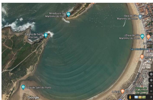
Figura 1: Devido à difração das ondas, as ondas do oceano que entram através de uma abertura natural podem se espalhar por toda a baía.
