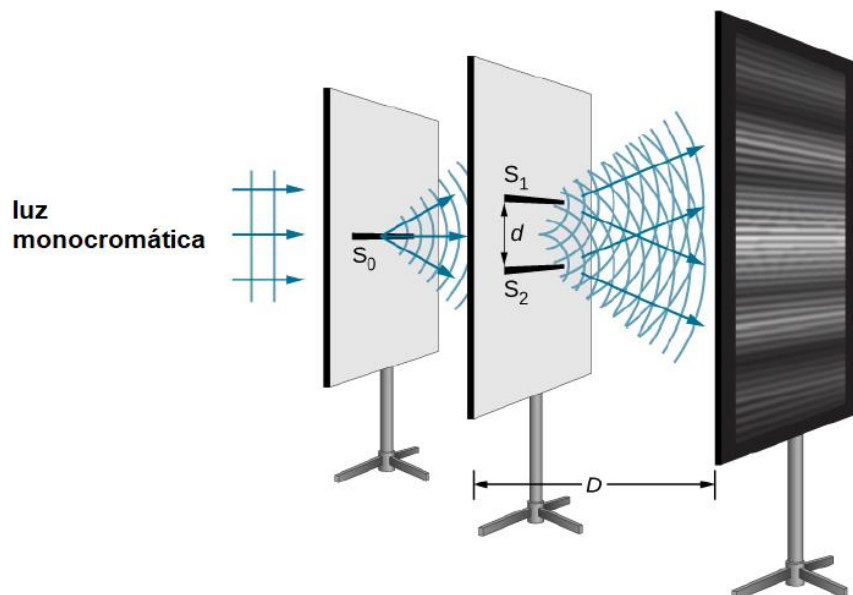
Figura 9 : O experimento de interferência de dupla fenda usando luz monocromática e fendas estreitas. Franjas produzidas pela interferência das ondas de huygens das fendas s_1 e s_2 são observadas na tela.
