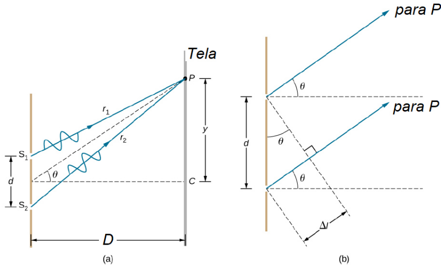
Figura 47: Esquema geométrico de duas ondas, representadas pelos raios r_1 e r_2 , passando através das fendas estreitas e interferindo no ponto p.
