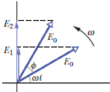
Figura 48: Fasores representando ondas.
