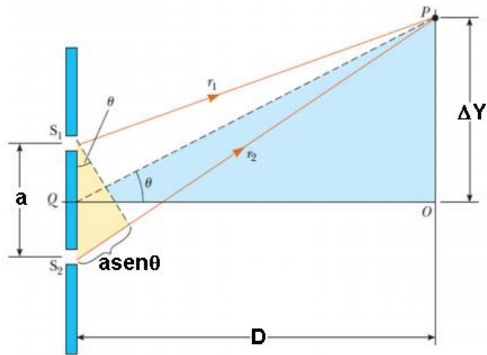
Figura 57: Difração entre duas fendas
