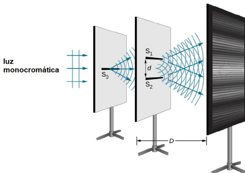
Figura 46 : O experimento de interferência de dupla fenda usando luz monocromática e fendas estreitas. Franjas produzidas pela interferência das ondas de Huygens das fendas s_1 e s_2 são observadas na tela.
