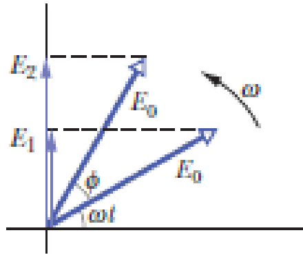
Figura 11: Fasores representando ondas.
