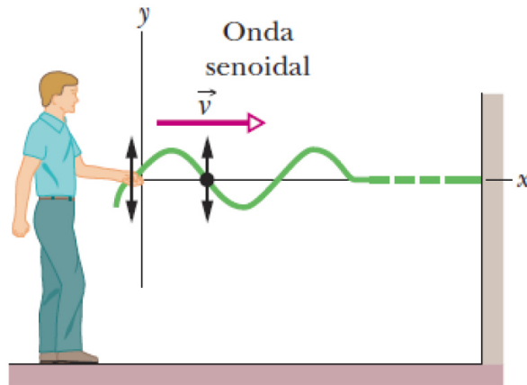
Figura 39 : Formação de uma onda numa corda.
