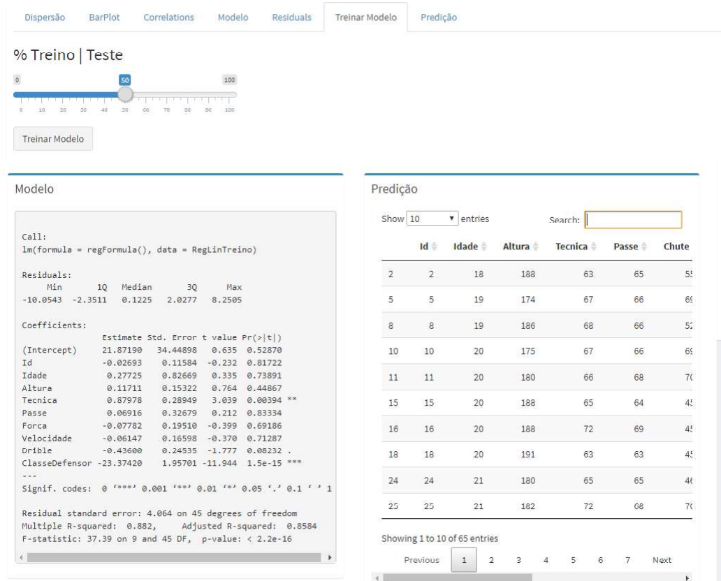
Figura 31 – Treino Regressão Linear
