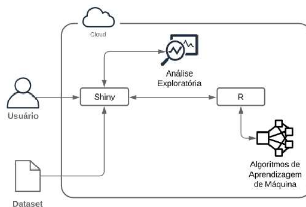
Figura 34 – Arquitetura da implantação na Nuvem
