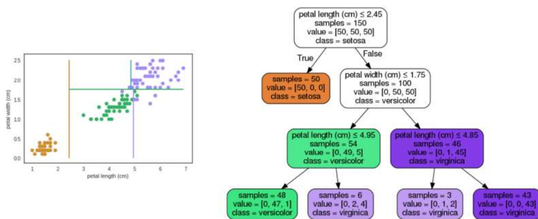
Figura 10 – Árvore de Decisão - Classificação
