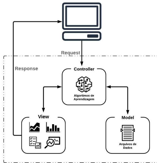
Figura 19 – Componentes MVC
