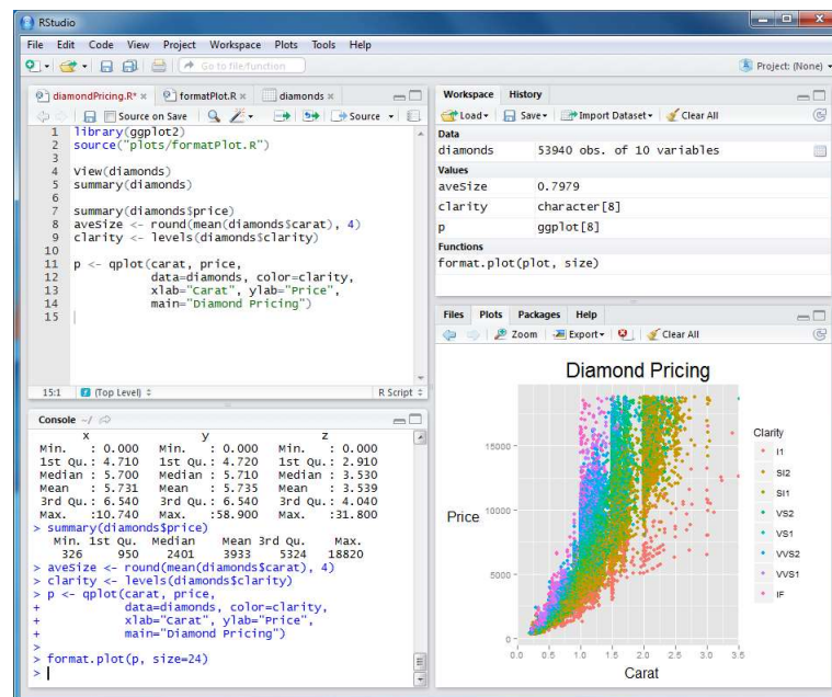
Figura 17 – RStudio
