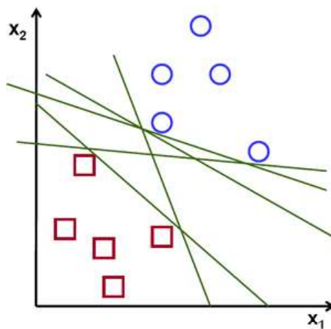
Figura 12 – Hiperplanos possíveis
