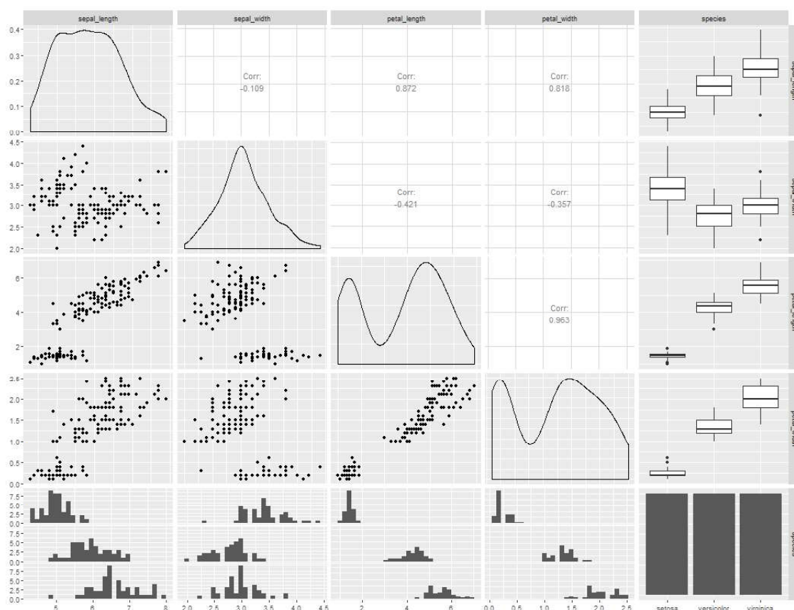
Figura 27 – Matriz de Correlação de Dados
