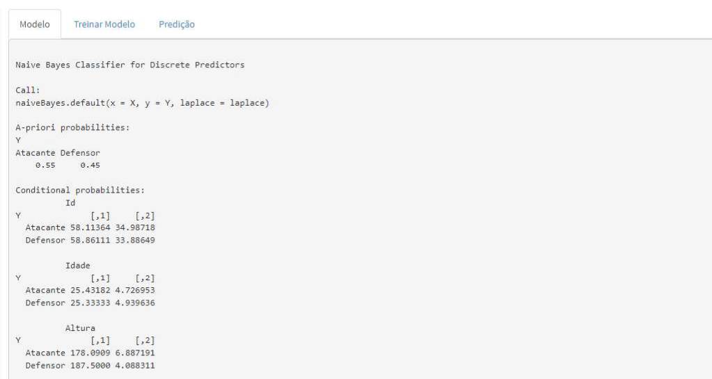
Figura 33 – Modelo de Classificação Naive Bayes com as opções de Treinar Modelo e Predição de novos valores
