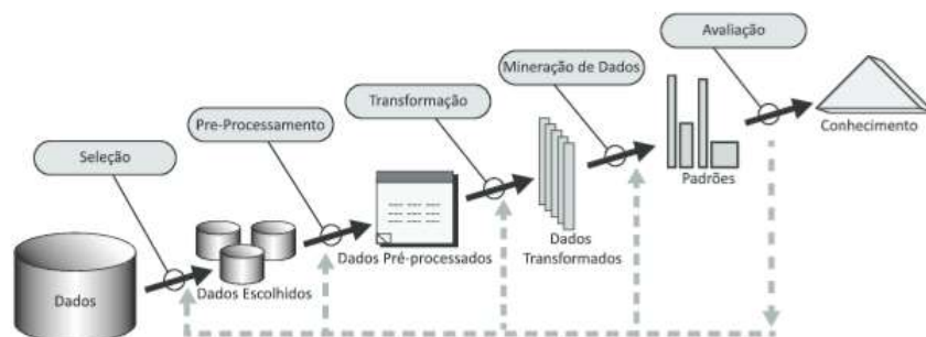
Figura 3 – Visão geral das etapas que constituem o processo KDD
