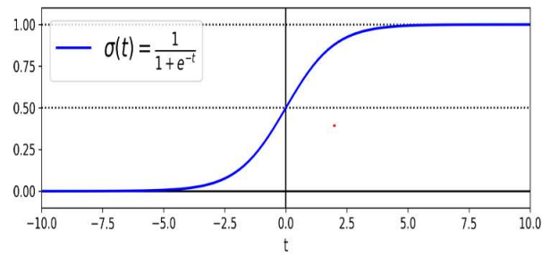
Figura 7 – Regressão Logística
