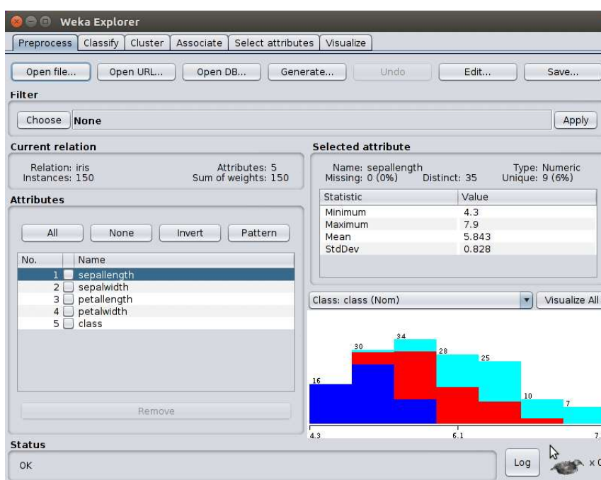
Figura 14 – Weka
