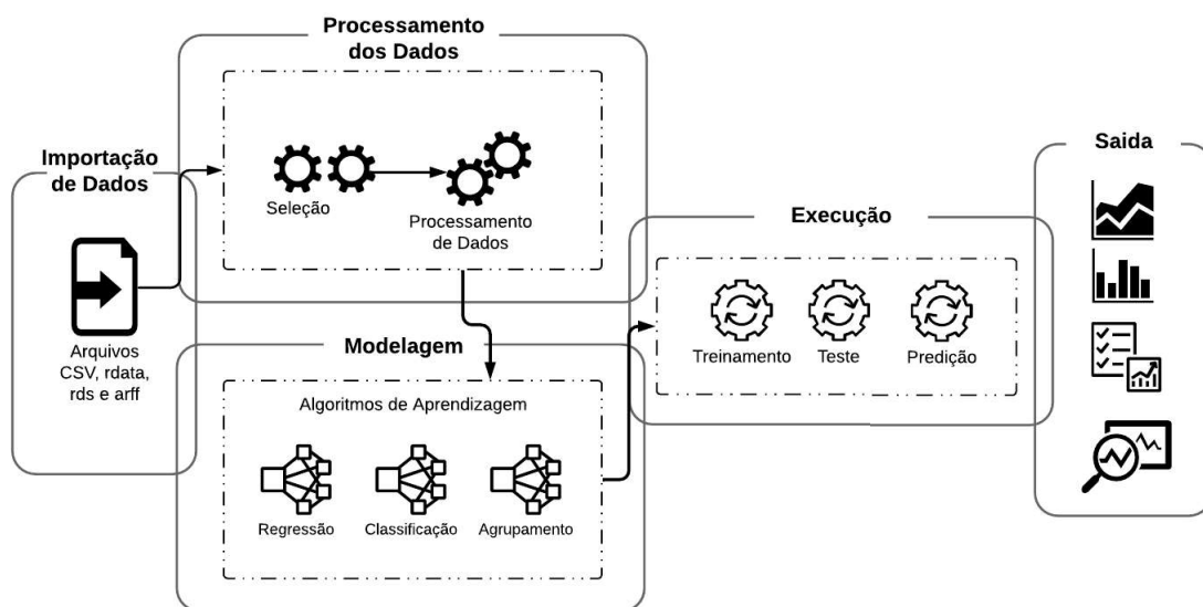
Figura 20 – Arquitetura LAWSMiner
