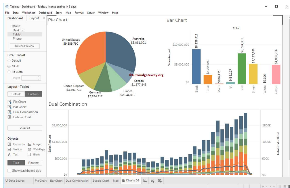
Figura 15 – Tableau
