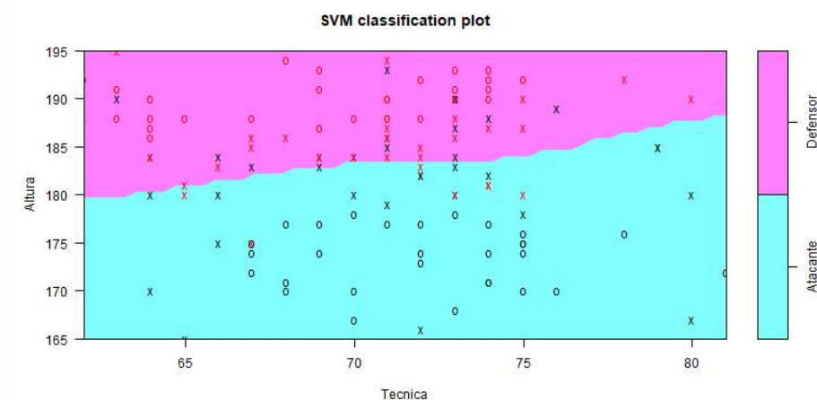
Figura 23 – Gráfico SVM. Classificação Classe tipo de jogador, nas dimensões de Altura e Técnica
