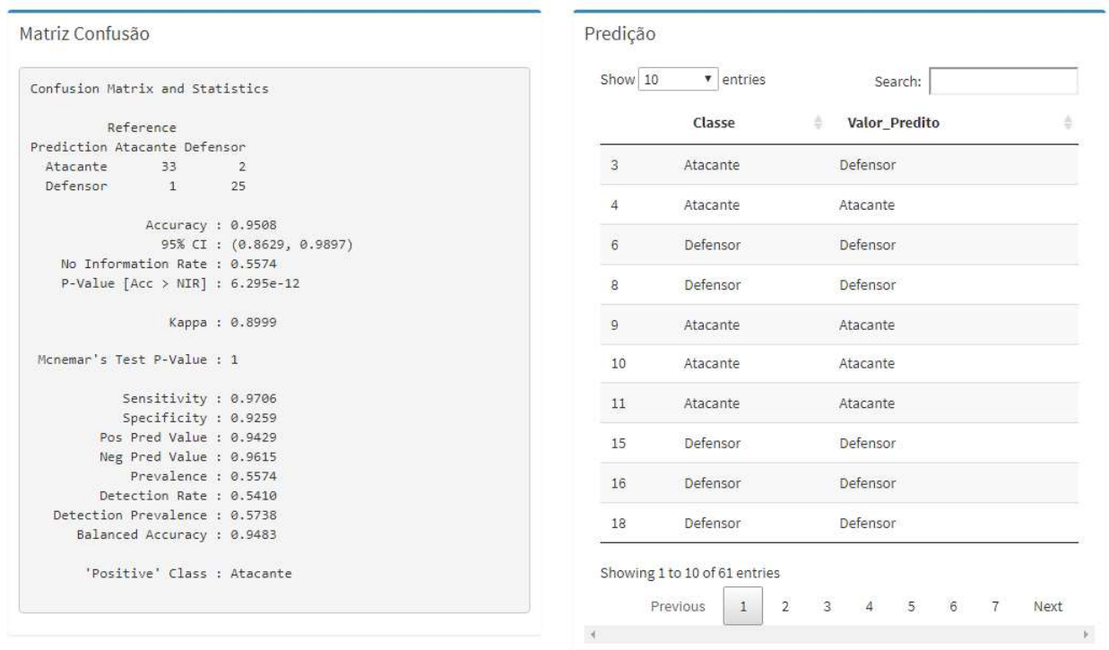
Figura 22 – Matriz Confusão e Predição do algoritmo Naive Bayes
