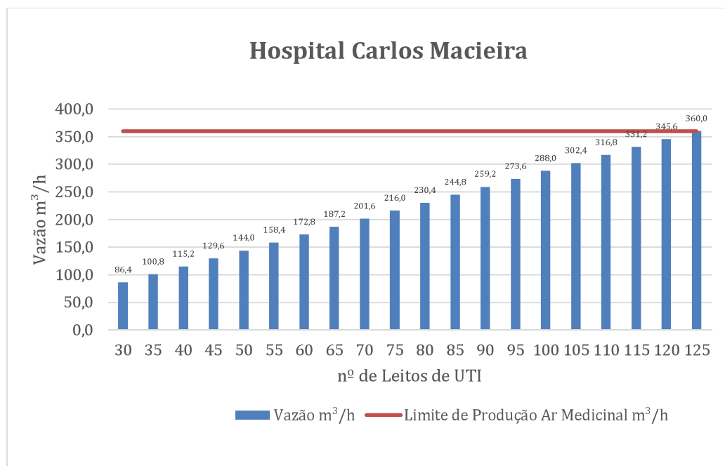
Figura 18 - Valores do Nº de Leitos x Vazão do Ar medicinal do Hospital Carlos Macieira (em m³/h) Fonte: do autor, 2025.
