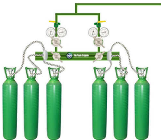
Figura 1. Central de suprimento com cilindros de oxigênio.
