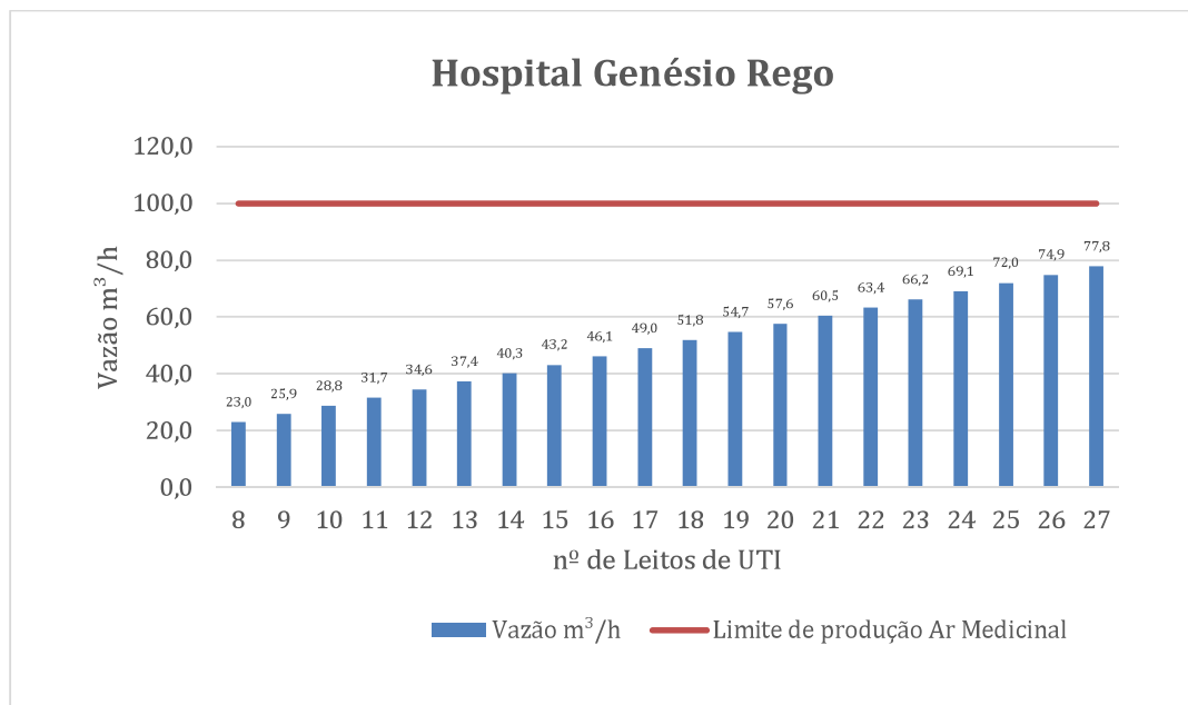
Figura 17 - Valores do Nº de Leitos x Vazão do Ar medicinal e gás oxigênio do Hospital Genésio Rego (em m³/h) Fonte: do autor, 2025.
