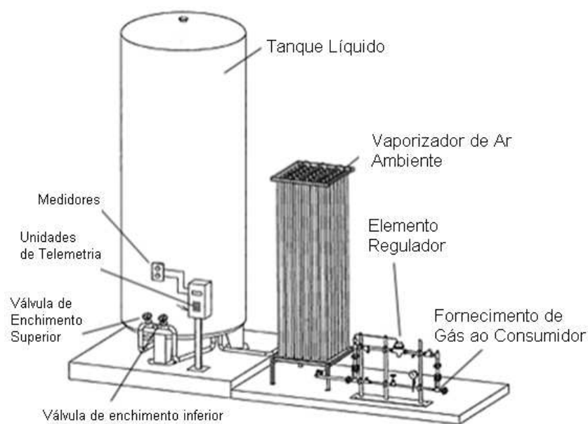
Figura 2. Sistema típico de armazenamento de oxigênio líquido juntamente com seção transversal do tanque de armazenamento.
