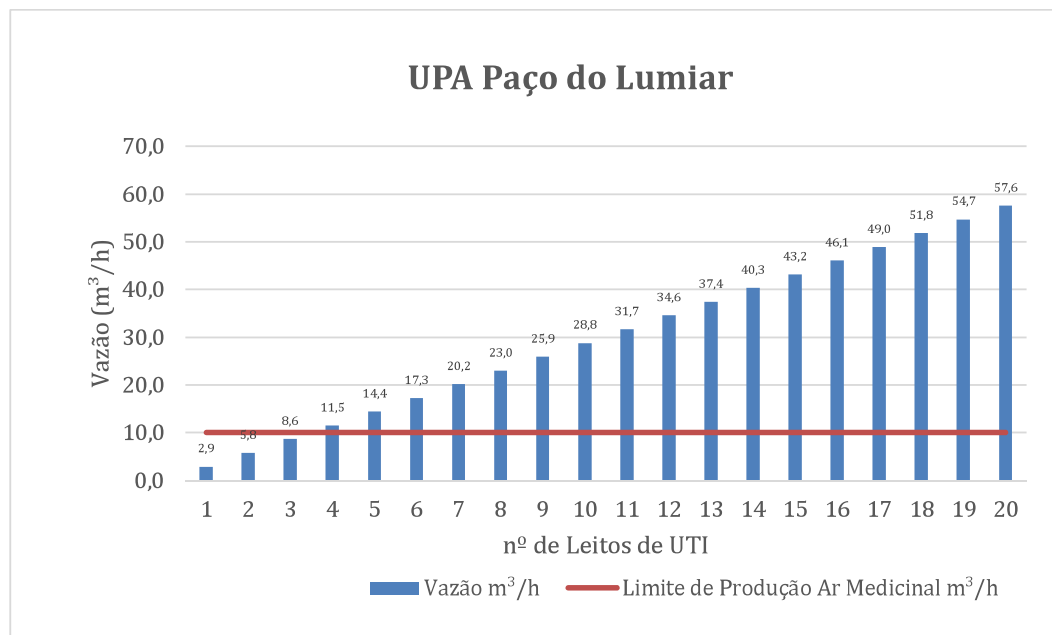
Figura 16 - Valores do N° de Leitos x Vazão do Ar medicinal e oxigênio da Unidade de Pronto Atendimento do Paço do Lumiar (em m 3 /h) Fonte: do autor, 2025.
