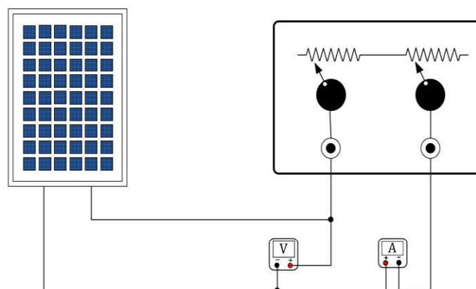
Figura 32-Conexão da placa na caixa 2 com resistores
