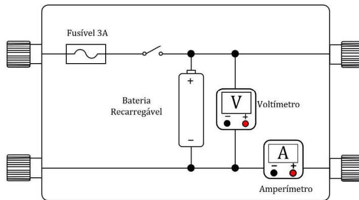
Figura 29-Caixa 1-bateria e Medidores
