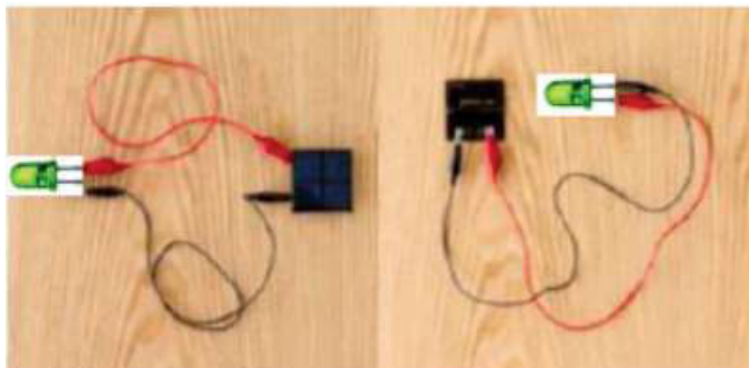
Figura 11 - Conexões mini-placa-led.
