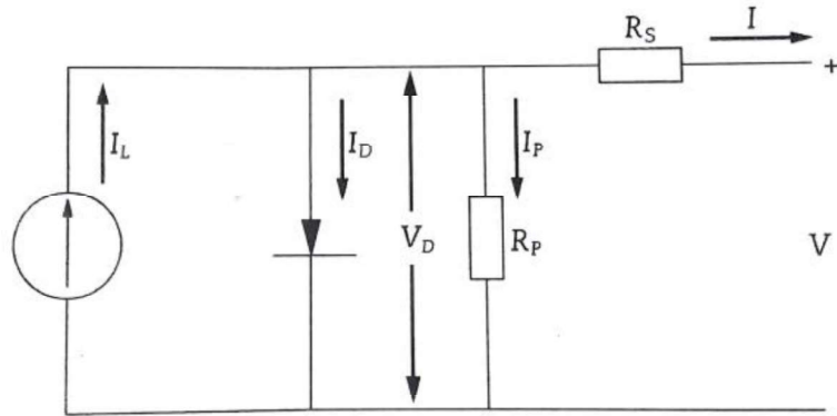
Figura 7-Circuito equivalente de uma célula fotovoltaica
