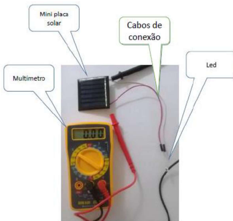
Figura 22-Circuito placa-led utilizada na SEI 02
