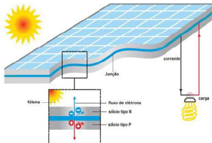
Figura 4-Representação do processo de conversão fotovoltaica
