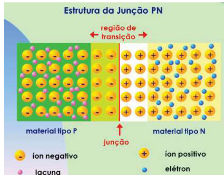
Figura 7 - Junção P-N.
