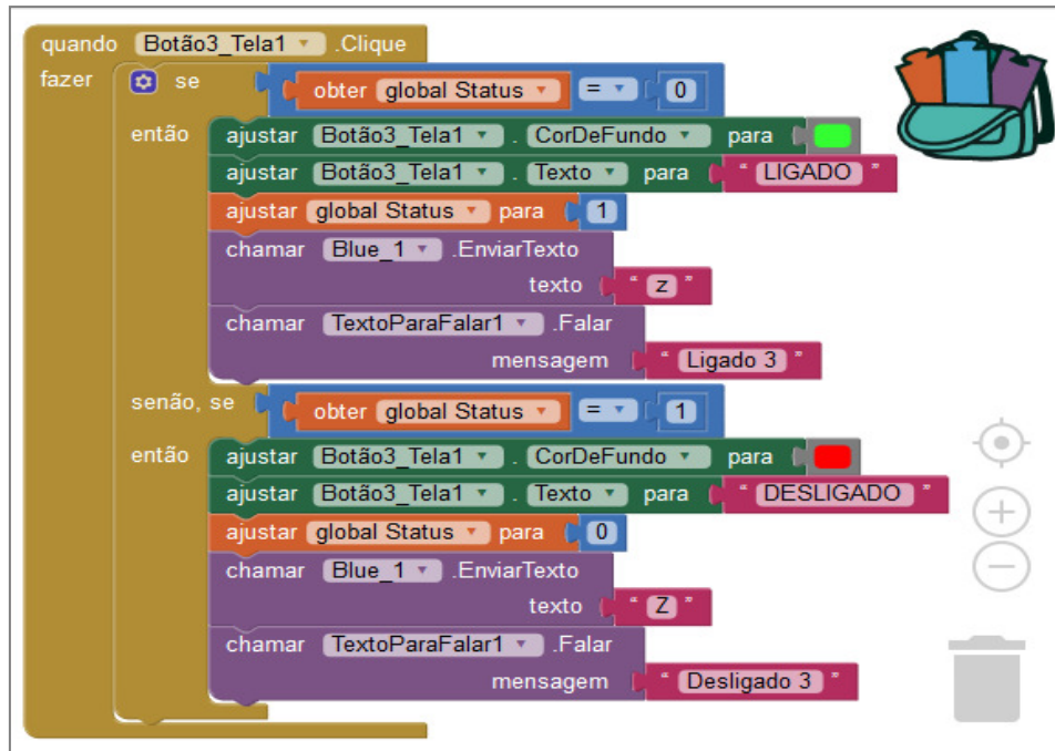
Figura 33 – Lógica de blocos do terceiro botão “Liga/Desliga”.
