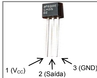
Figura 86 - Sensor de temperatura LM35.
