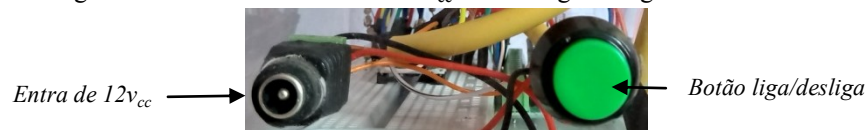
Figura 98 – Entrada de fonte de 12V cc e botão liga/desliga do Eletrouino.
