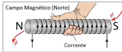
Figura 92 – Regra da mão direita para o solenoide.
