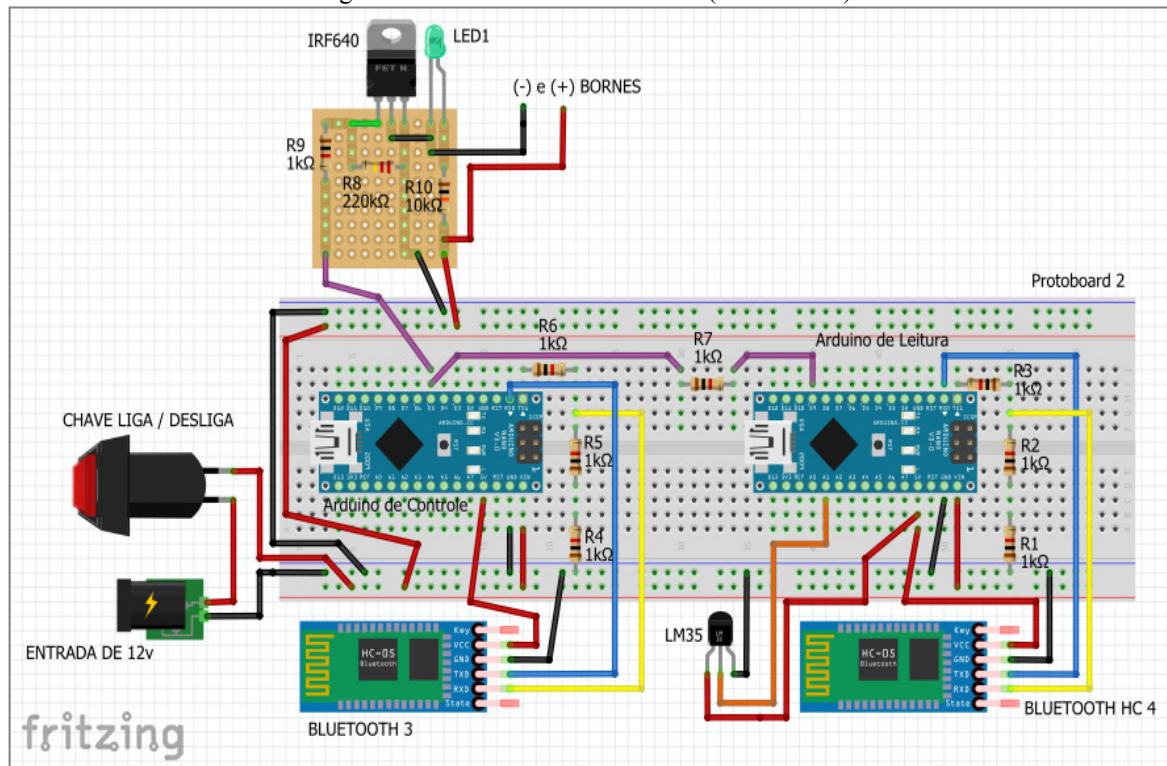
Figura 85 – Circuito do Eletroduino (Efeito Joule).
