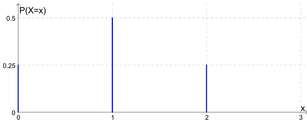
Figura 2.2: Distribuição de probabilidade de uma v.a. X = número de coroas em dois lançamentos de uma moeda honesta.
