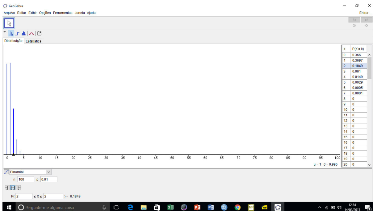
Figura 4.16: Distribuição de probabilidade da v.a. X \sim B(100; 0,01) .
