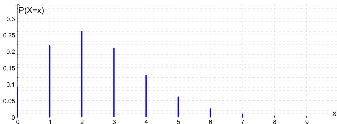
Figura 4.4: Distribuição de Poisson com média \alpha = 2,41 .
