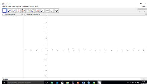
Figura 4.5: Tela inicial do GeoGebra.
