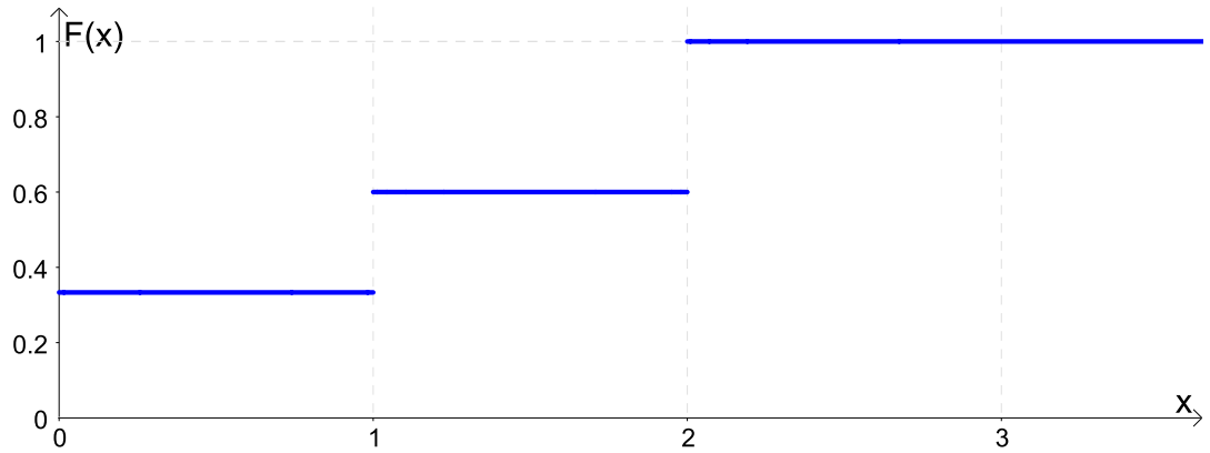
Figura 2.3: Representação gráfica de uma função de distribuição acumulada de uma v.a. discreta.
