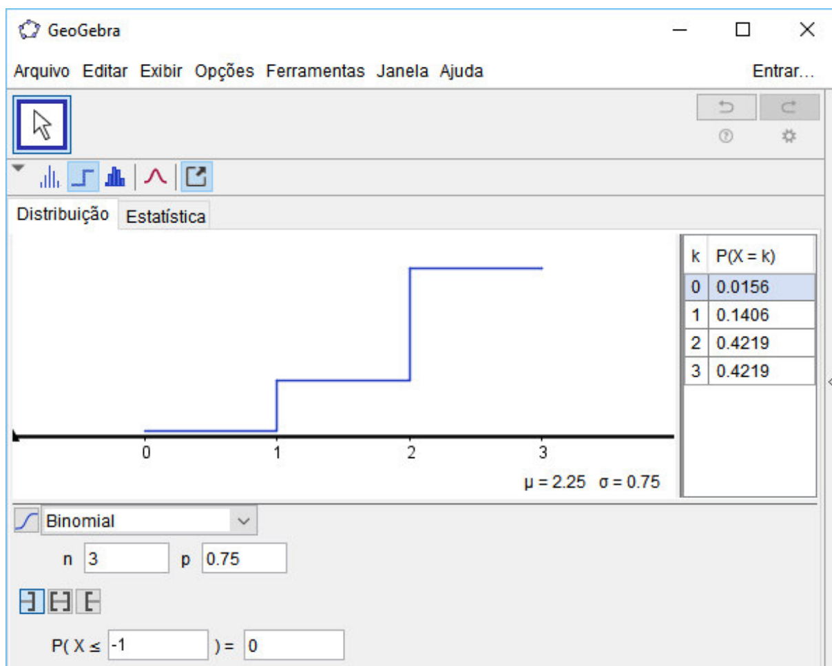
Figura 4.14: Probabilidade de X para valores menores que zero na Aplicação 4.5.
