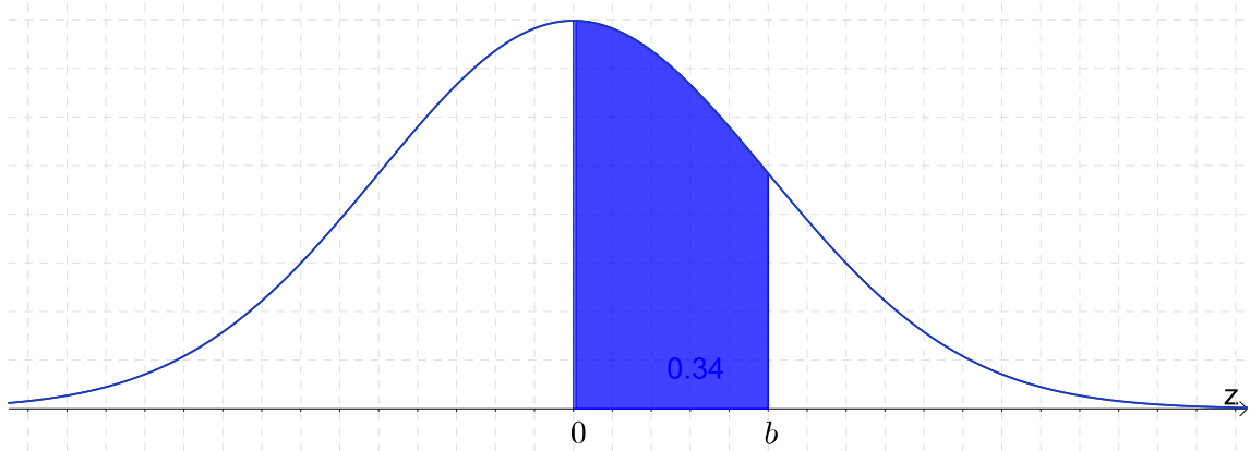
Figura 2.9: P(0 \leq Z \leq b) representada pela área sombreada para b fixado.
