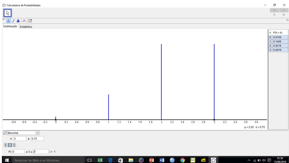
Figura 4.12: Gráfico da distribuição de probabilidade da v.a. X \sim B(3; 0,75) .
