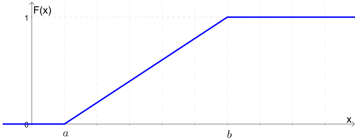
Figura 2.5: Modelo gráfico da fd de uma v.a. X \sim U[a, b] .
