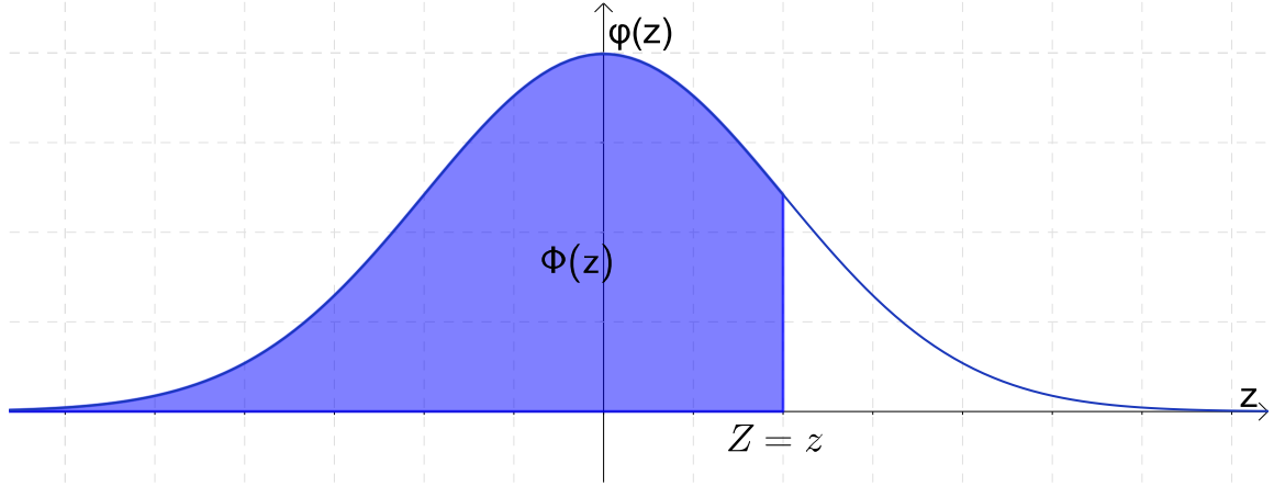
Figura 2.8: \Phi(z) = P(-\infty < Z \leq z) representada pela área sombreada.
