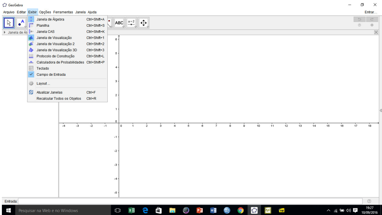
Figura 4.7: Localização da calculadora de probabilidade no GeoGebra.
