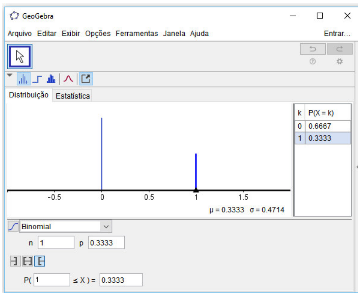
Figura 4.15: Distribuição de Bernoulli.
