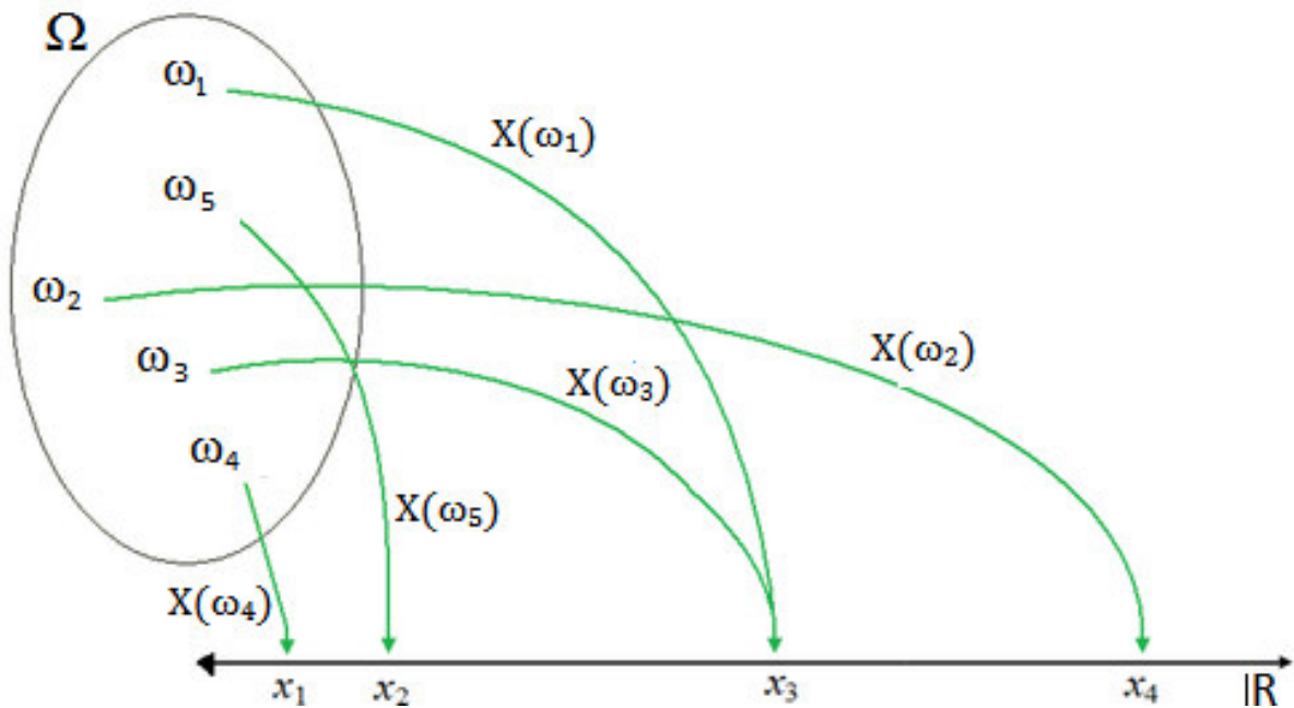
Figura 2.1: Representação esquemática de uma variável aleatória X .
