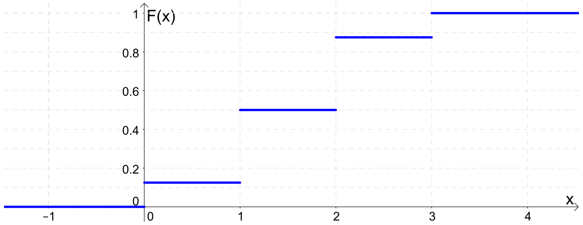
Figura 3.2: Gráfico da distribuição acumulada da v.a. X \sim B(3; 0,5) do Exemplo 3.1.
