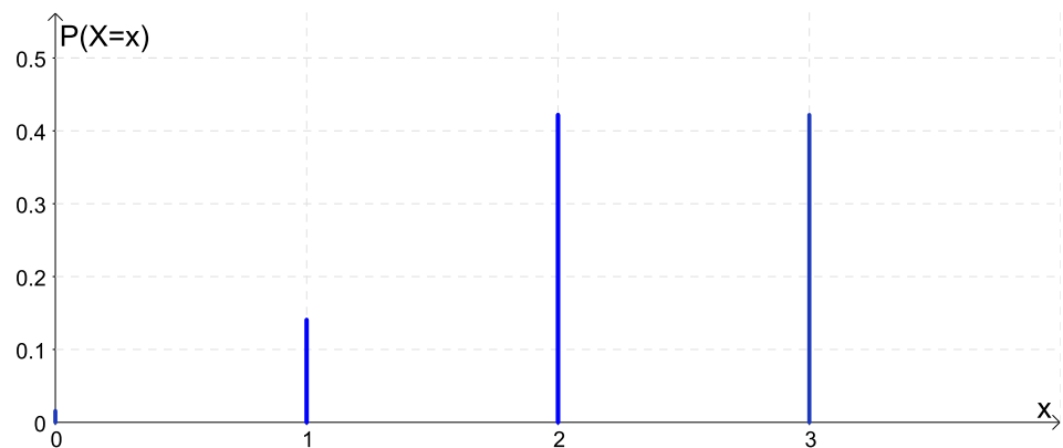
Figura 4.10: Gráfico da função de distribuição de probabilidade da v.a. X \sim B(3; 0,75) .
