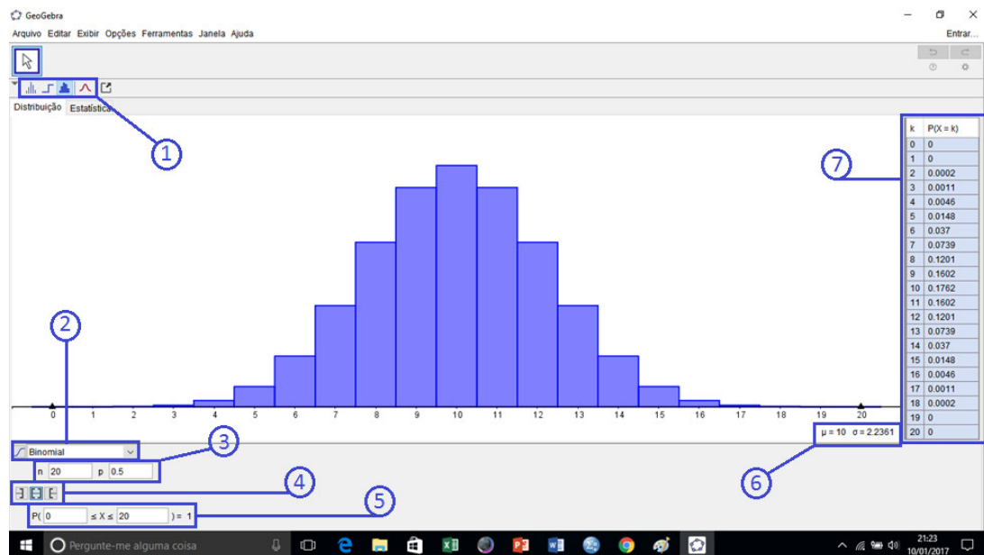
Figura 4.8: Calculadora de probabilidade mostrando a função de probabilidade da v.a. X \sim B(20; 0,5) .
