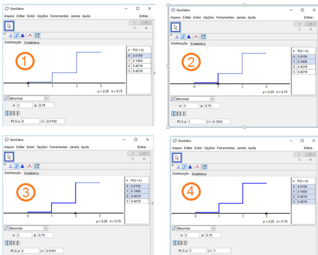
Figura 4.13: Representação gráfica da função de distribuição acumulada de X \sim B(3; 0, 75) .
