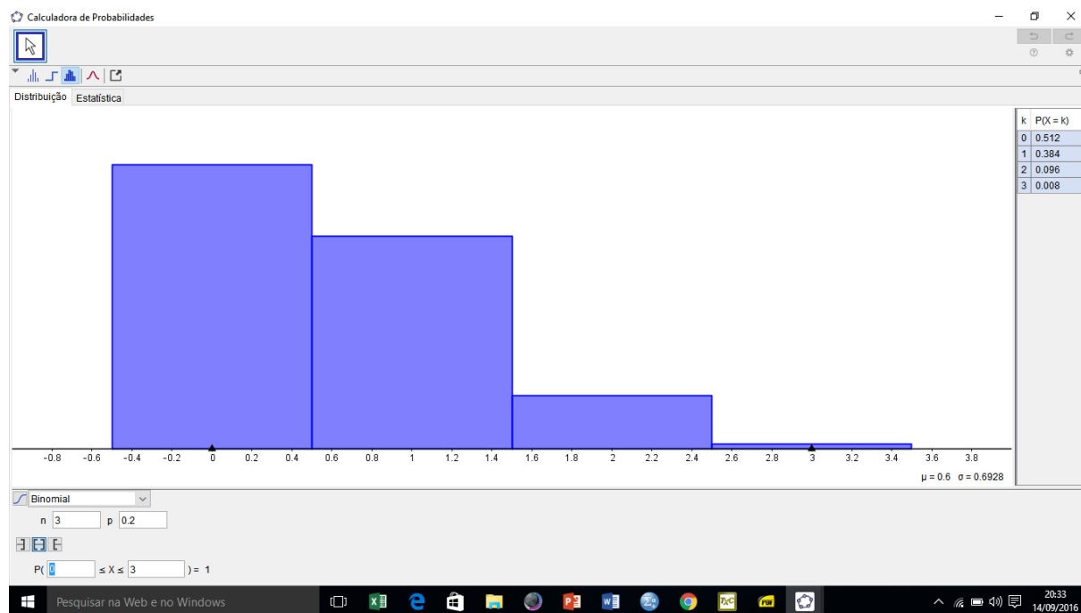
Figura 4.9: V.a. X distribuída binomialmente com parâmetros (3; 0, 2) .
