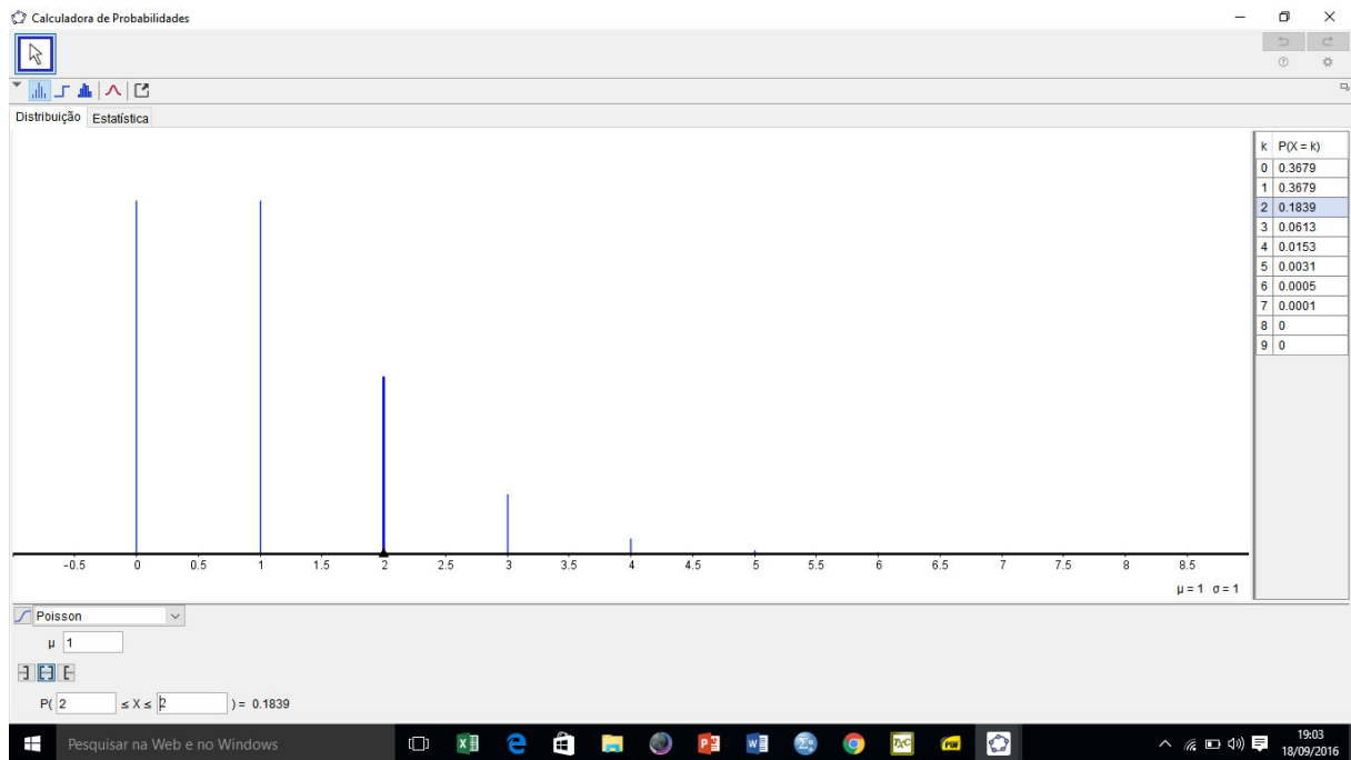
Figura 4.17: Distribuição de Poisson com \alpha = 1 .
