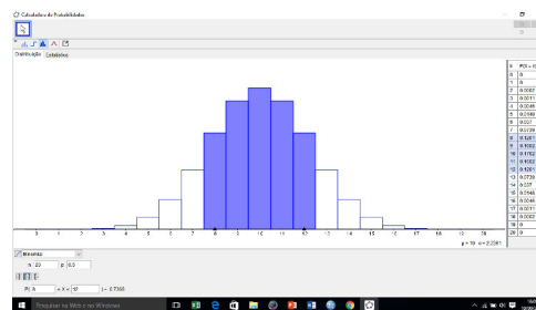
Figura 4.6: Calculadora de probabilidade do GeoGebra.
