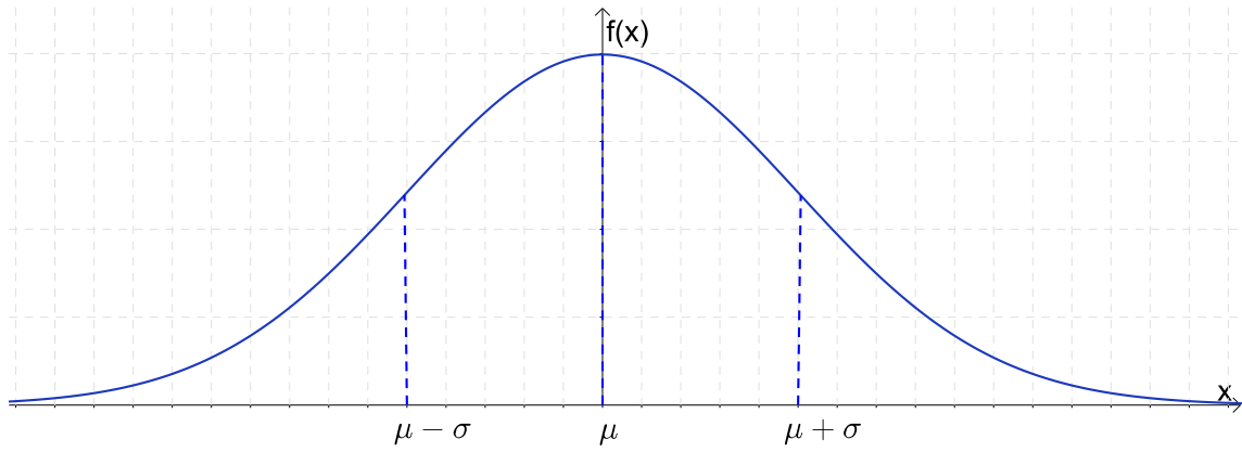
Figura 2.7: Representação gráfica da f(x) da v.a. X \sim N(\mu, \sigma^2) .
