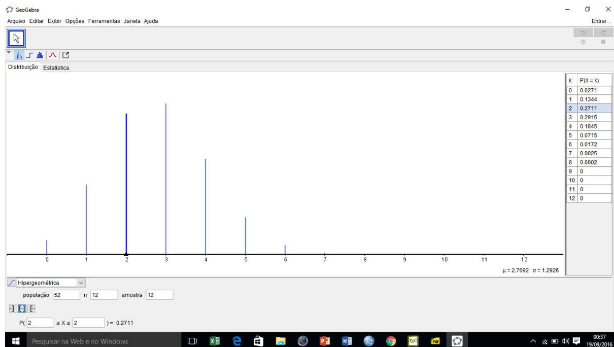
Figura 4.18: Distribuição hipergeométrica.
